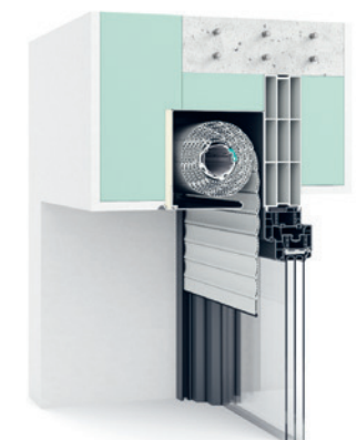
Putzträgerkasten. Rollgeformte Blenden. Vorder- und Revisionsblende aus stranggepresstem Aluminium in Ausführung 90°.
