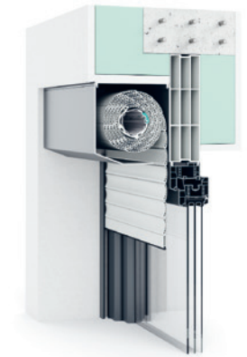
Vorbaukasten Standard. Rollgeformt oder stranggepresst in abgeschrägter Ausführung 20°.
