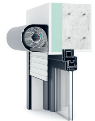
Rundkasten. Rollgeformt oder stranggepresst in runder Ausführung.
